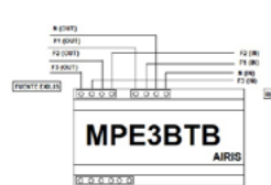
Conexionado Módem trifásico
